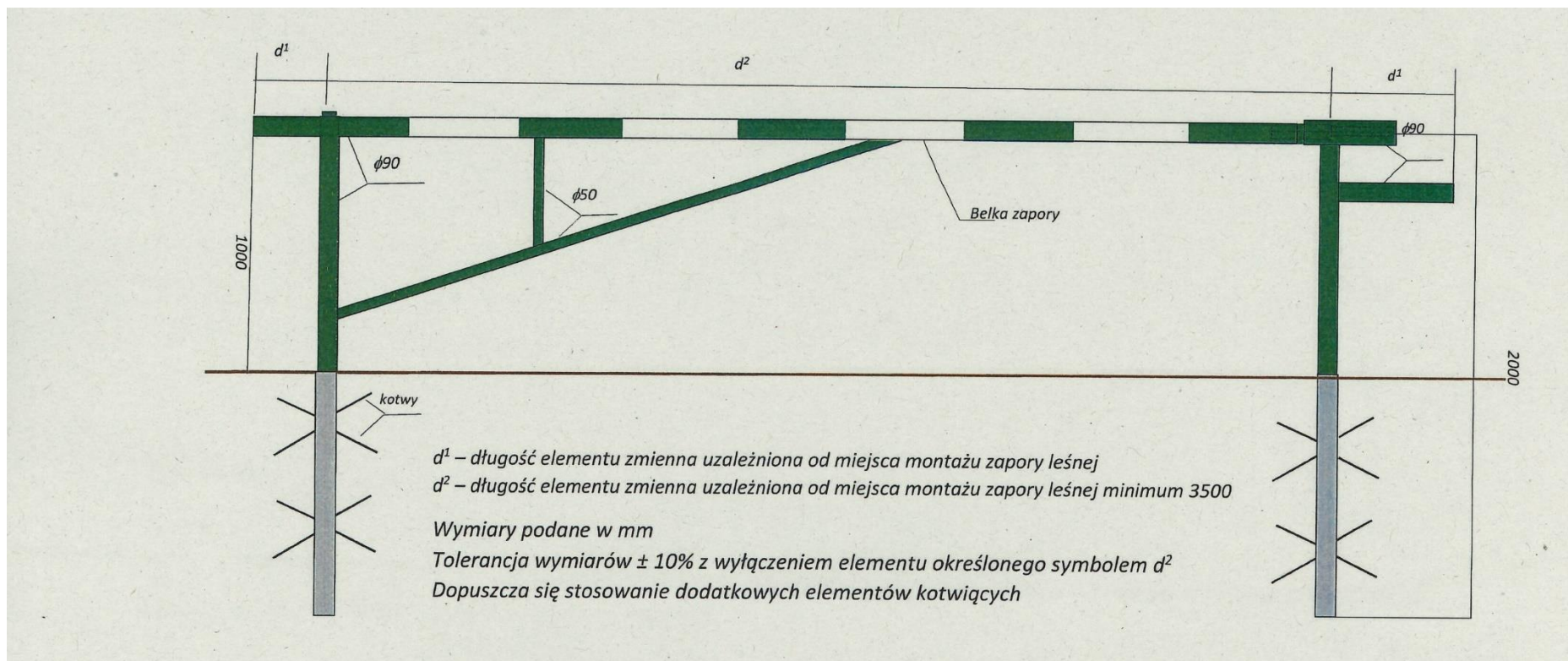
Ryc.5 Rysunek podglądowy zapory leśnej wraz z parametrami (źródło: Zarządzenie nr 36 Dyrektora Generalnego Lasów Państwowych z dnia 28 maja 2021 r., załącznik nr 5)
