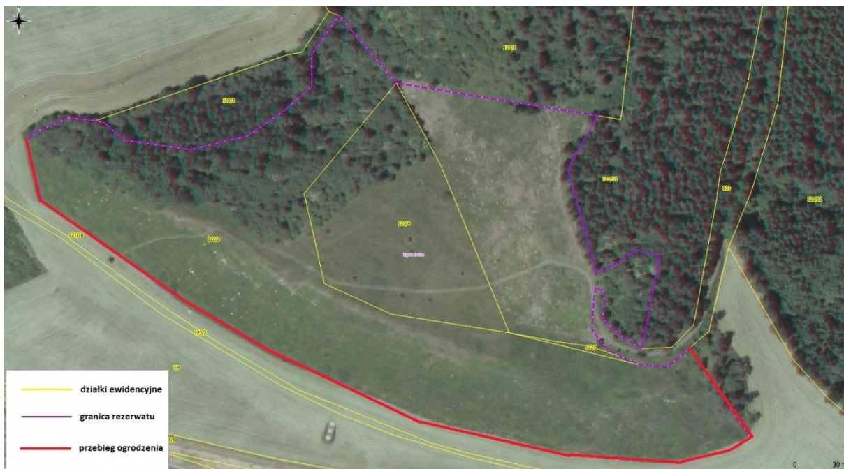
Ryc. 1. Orientacyjna lokalizacja elementów ogrodzenia - przebieg wzdłuż południowej granicy działki
