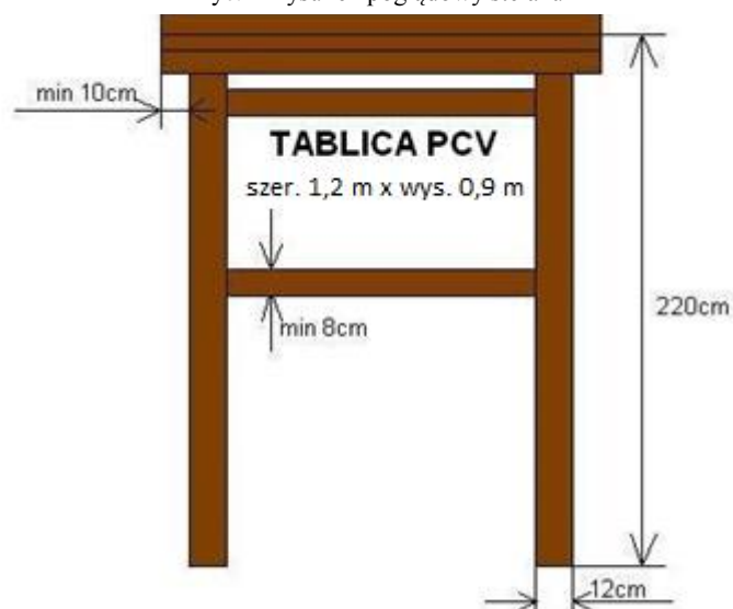
Ryc. 1 Rysunek poglądowy stelażu
